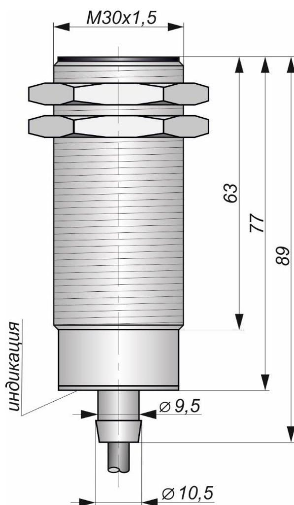
Габаритный чертеж
